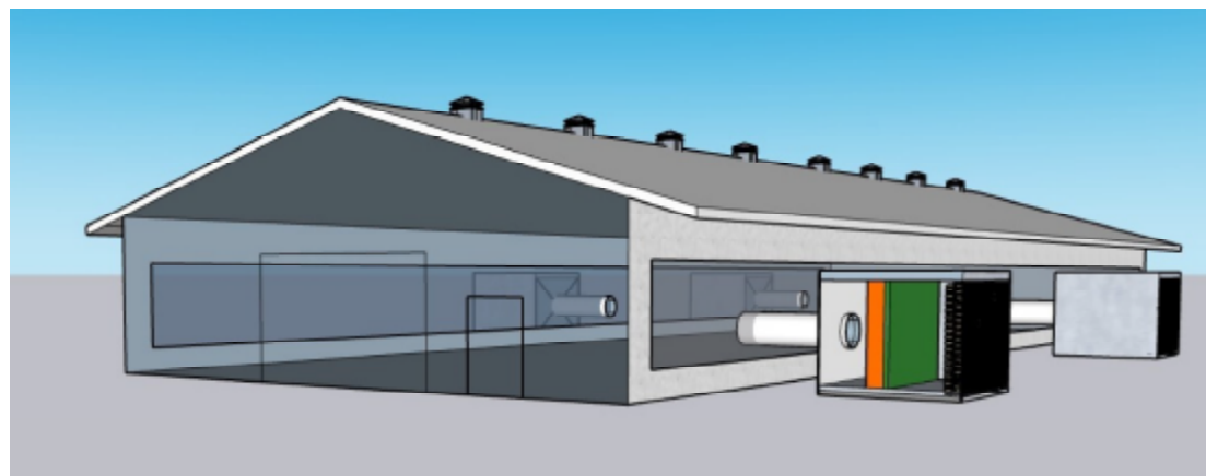
Grafik 45: Stall mit außen angebrachtem Überdrucksystem mit geschlossenen Jalousien
